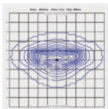
CORBES ISOLUX UNITÀRIES
