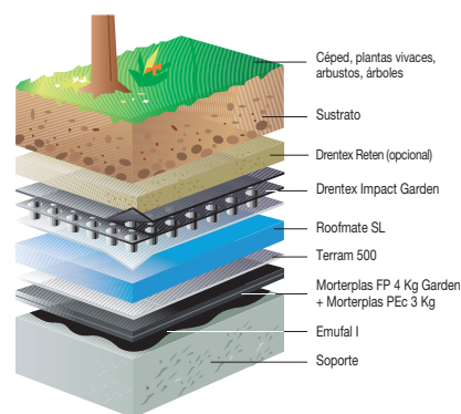
■ Ejemplo cubierta ajardinada intensiva invertida
