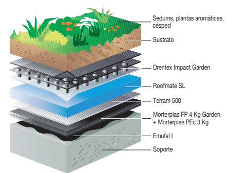
■ Ejemplo cubierta ajardinada extensiva invertida
